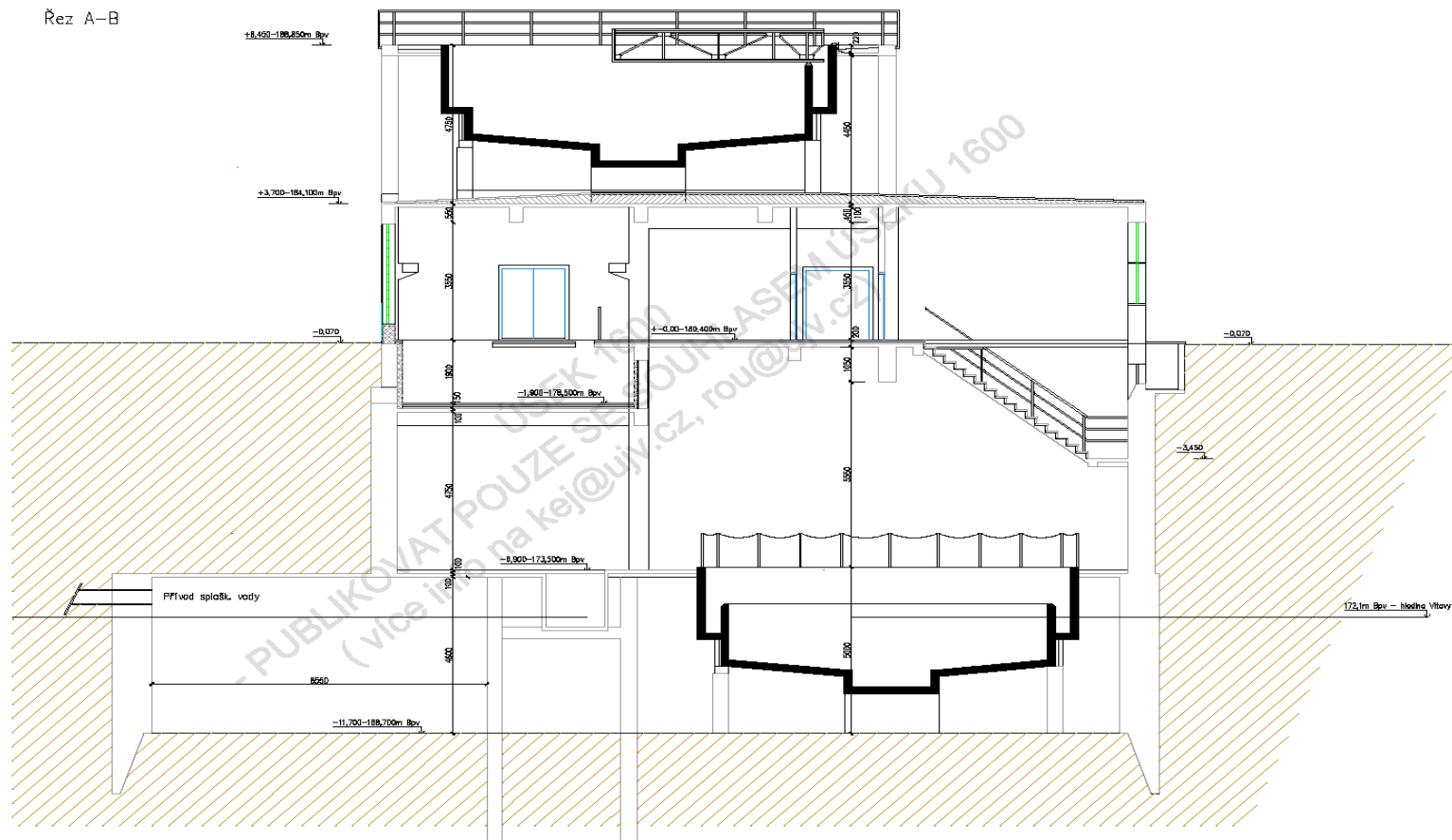
Řez A-B
