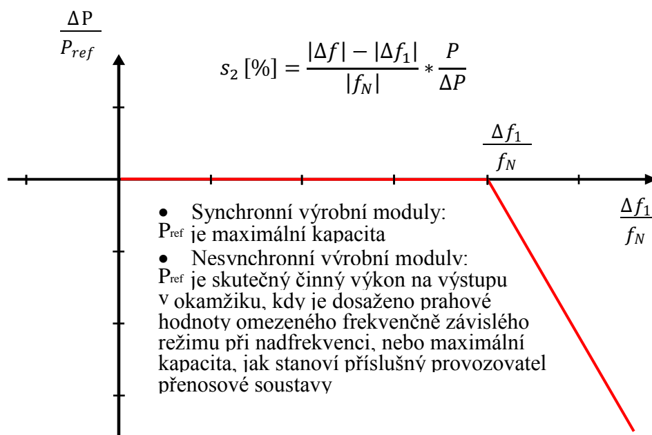
Obr. 5 - Schopnost frekvenční odezvy činného výkonu u výrobních modulů v omezeném frekvenčně závislém režimu při nadfrekvenci
