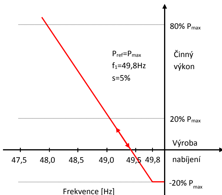
Obr. 7 - Frekvenční odezva činného výkonu na podfrekvenci u akumulárního zařízení
