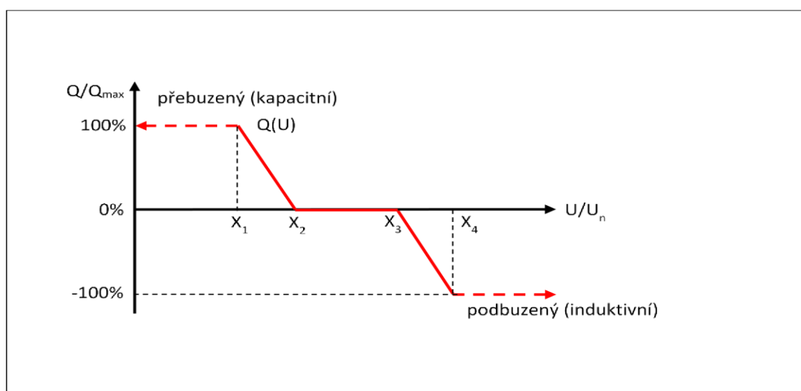
Obr. 9 - Charakteristika funkce Q(U)
