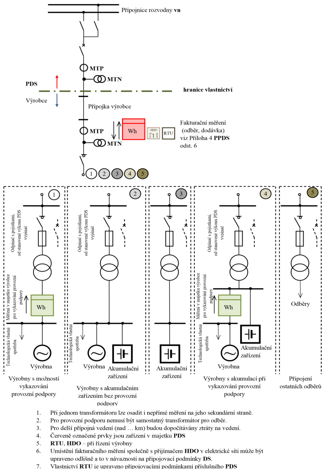
Obr. 13 - Připojení výroby a akumulačního zařízení samostatným vedením do vn rozvodny DS
