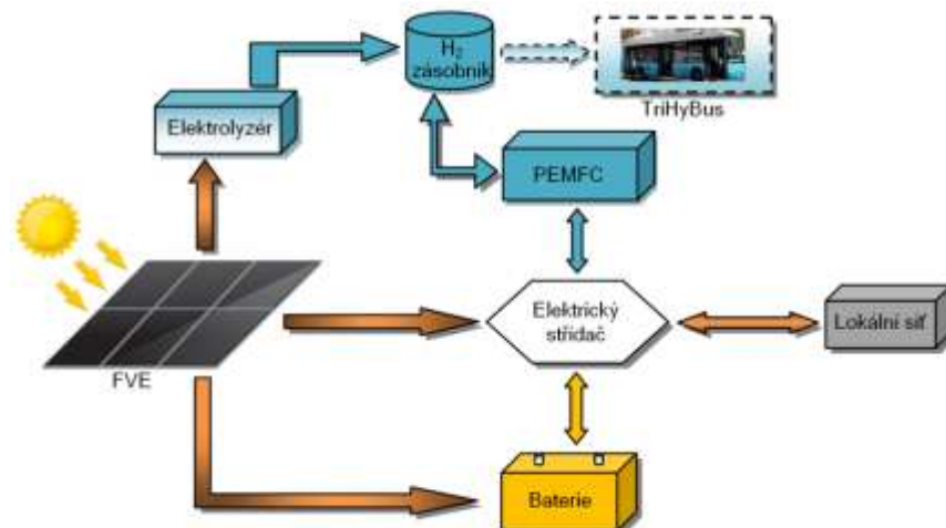
Schéma propojení fotovoltaických panelů a vodíkového akumulacího systému
